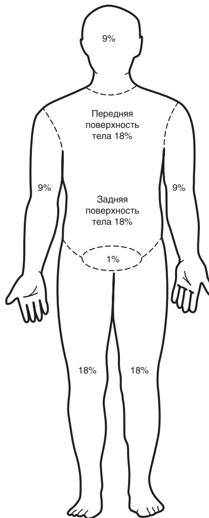
Рис. 21.3. Правило девяток
